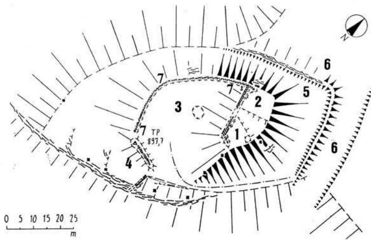
Grundriß von Boris Blum, Lauben 1992.
