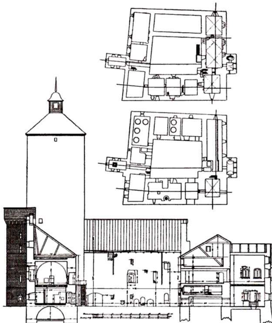
Querschnitt des West- und Ostflügels der Hauptburg. Grundriss des 1. und 2. Stockwerkes, nach Karling
